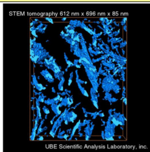
写真 「Cellmapp」を用いて作製した CNF/PP(=3:97)複合材料のSTEM tomography 画像 (612nm x 696nm x 85nm) UBE科学分析センター様から御提供
