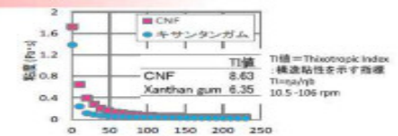
(図1) CNF及びキサンタンガムの粘度測定(各0.8wt%)
